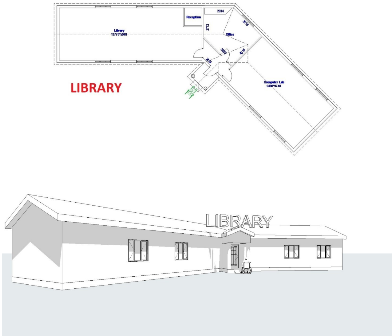
Bauplan des «Connect and Learning Center» mit Bibliothek und Computerraum, inklusive Empfangsraum und Büro.
